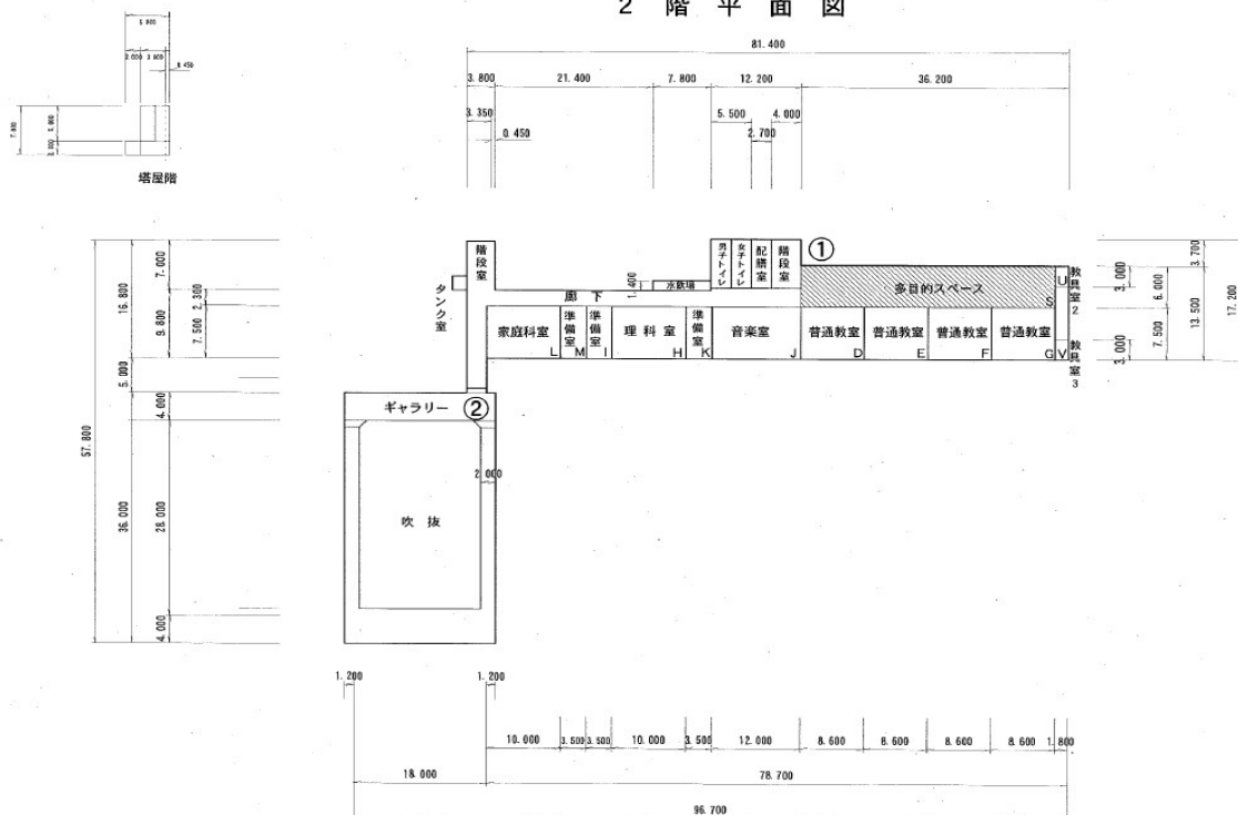
2 階 平面図
