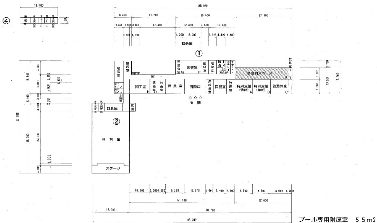
1 階 平面図
