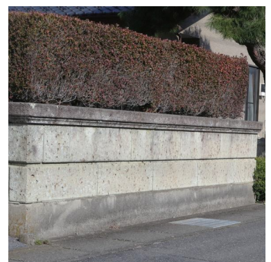
健全な石塀
